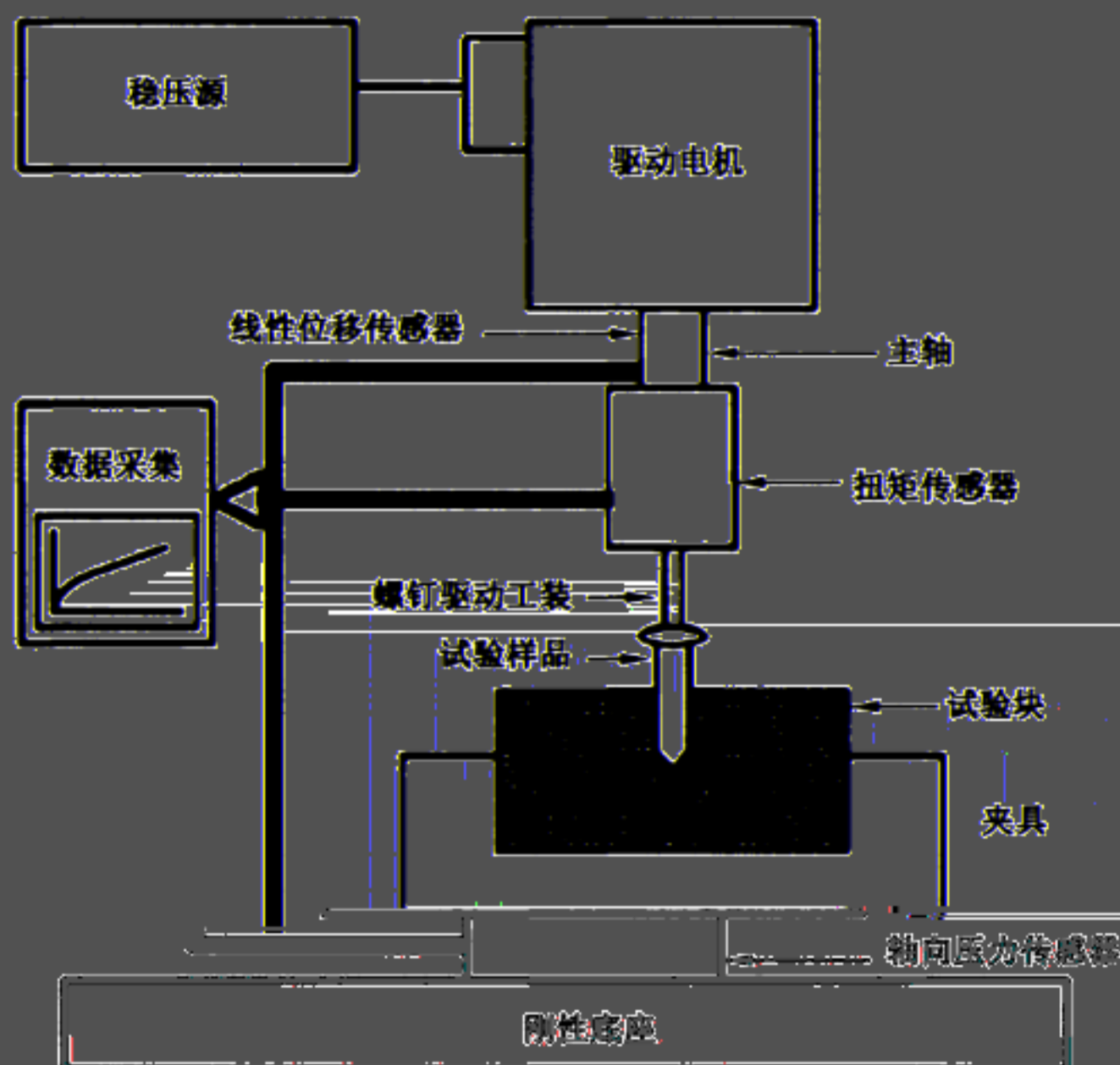
图1 自攻性能试验装置
